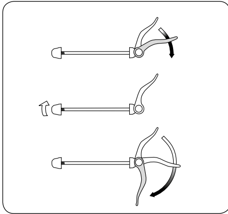
Einstellmutter lösen
