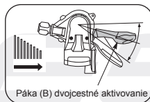
Prepnutie z veľkého na menší ozubený veniec (páka B)
