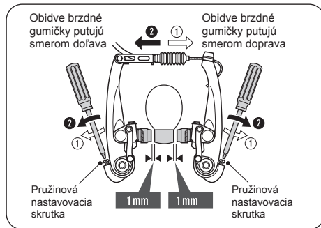
Nastavenie brzd na ráfiku
