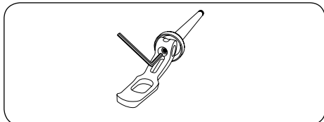
Átütőtengely beállítása gyorsrögzítő karral inbuszkulccsal
